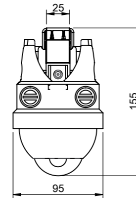
M7: Earth-Serie, Opto-Serie (Aufbauehäuse)
