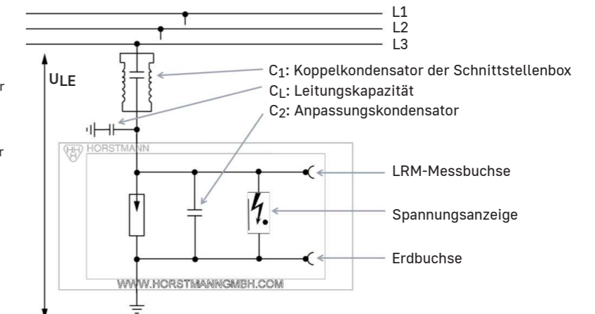
Prinzip des integrierten kapazitiven Spannungsprüfers für Niederspannungsanwendungen
