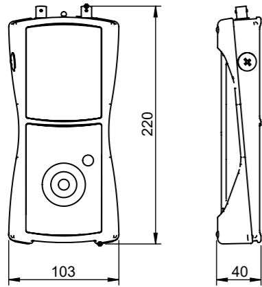
M16: Orion 3.1, Orion M1
