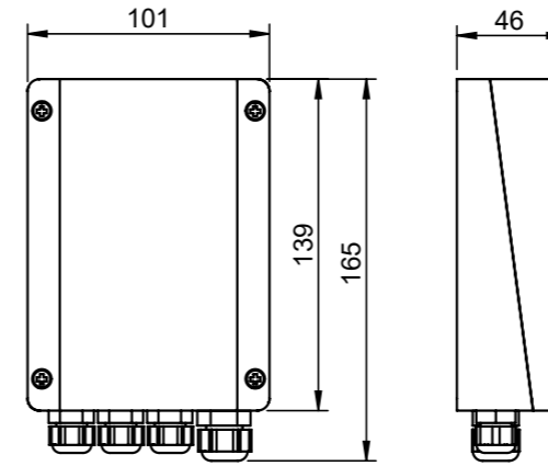
M7: Earth-Serie, Opto-Serie (Aufbauehäuse)
