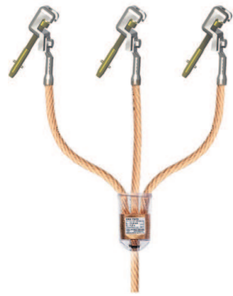
Phasenseitig mit Kugelzange
