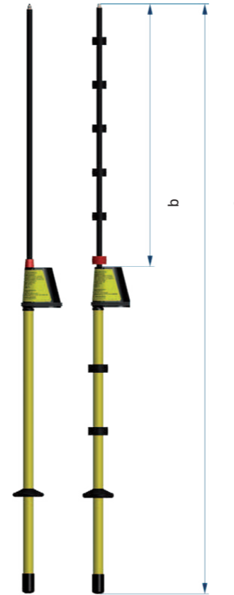
Comet BL-I | Comet BL-A mit Anzeigeeinheit
