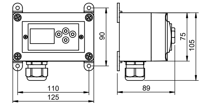
M13: Wega T1
