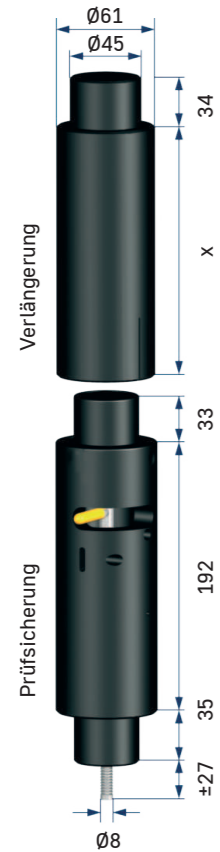
Prüfsicherung mit Verlängerung
