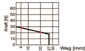
Prüfsicherung mit Verlängerung
