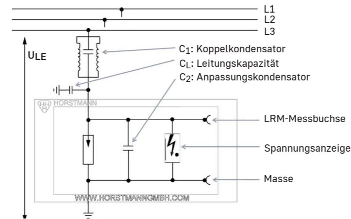
Prinzip des integrierten kapazitiven Spannungsprüfers
