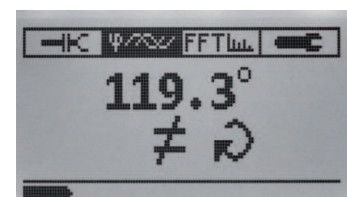
Anzeige Phasenvergleich
