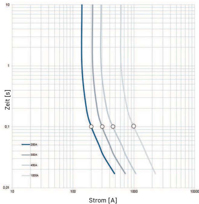
Strom- / Zeit-Kennlinie
